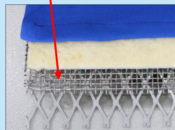
檯板結構 Table top structure
