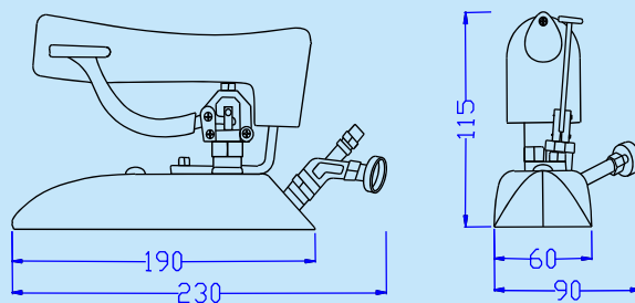
熨鬥尺寸簡圖 Iron Dimensions Diagram (mm)
